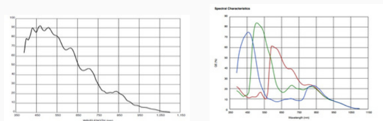
MV-CE050-30UM/UC
